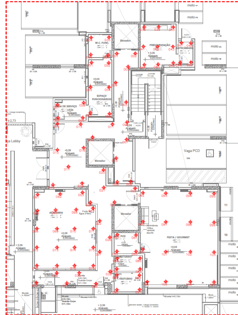
PLANTA DE MAPEAMENTO — TÉRREO
