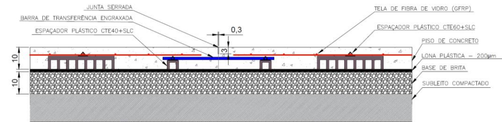
DETALHE DE JUNTA SERRADA SEM ESCALA
