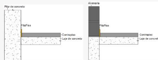
Figura 1 – Juntas de dessolidarização do contrapiso com argamassa autoadensável na interface com pilares e alvenarias
