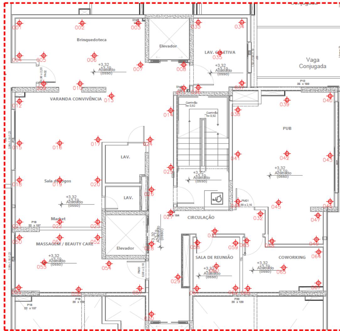
PLANTA DE MAPEAMENTO — MEZANINO
