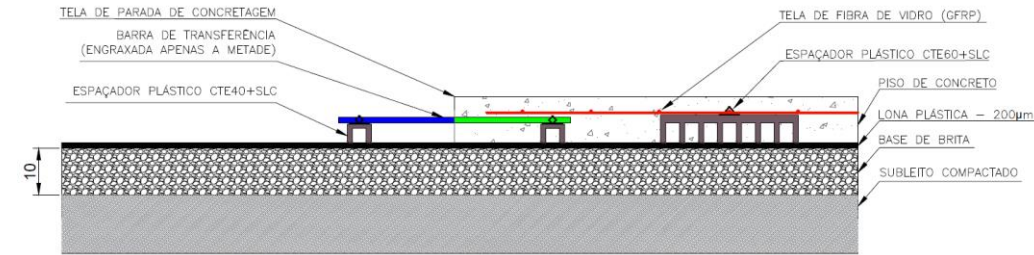
DETALHE DE JUNTA CONSTRUTIVA SEM ESCALA
