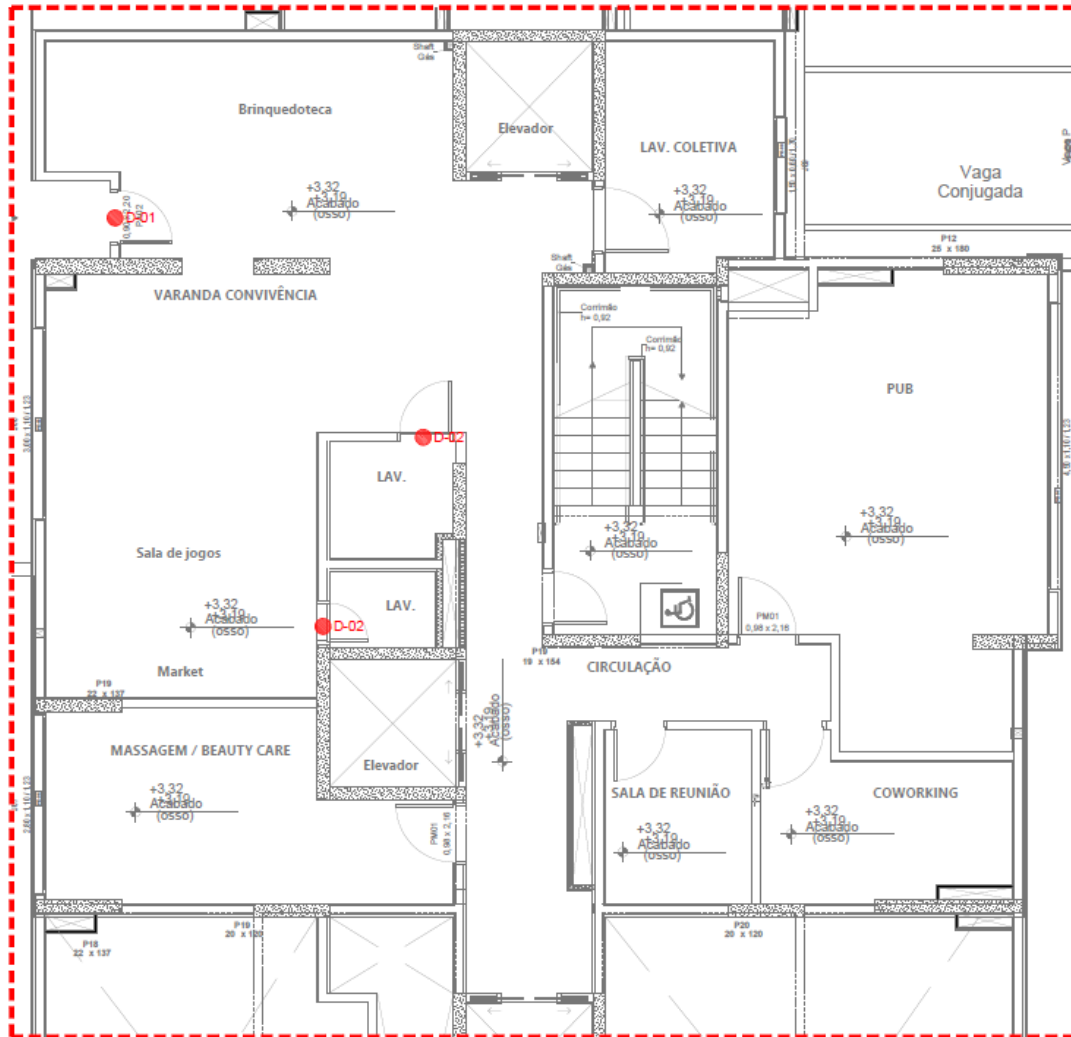
PLANTA DE DETALHES DE INTERFACE – MEZANINO
