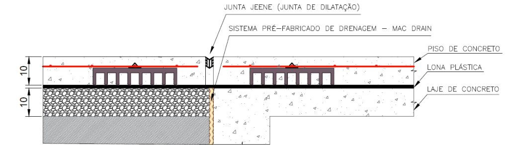
DETALHE DE JUNTA DE DILATAÇÃO SEM ESCALA
