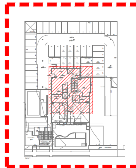
PLANTA DE CONTRAPISO – PAVIMENTO TIPO
